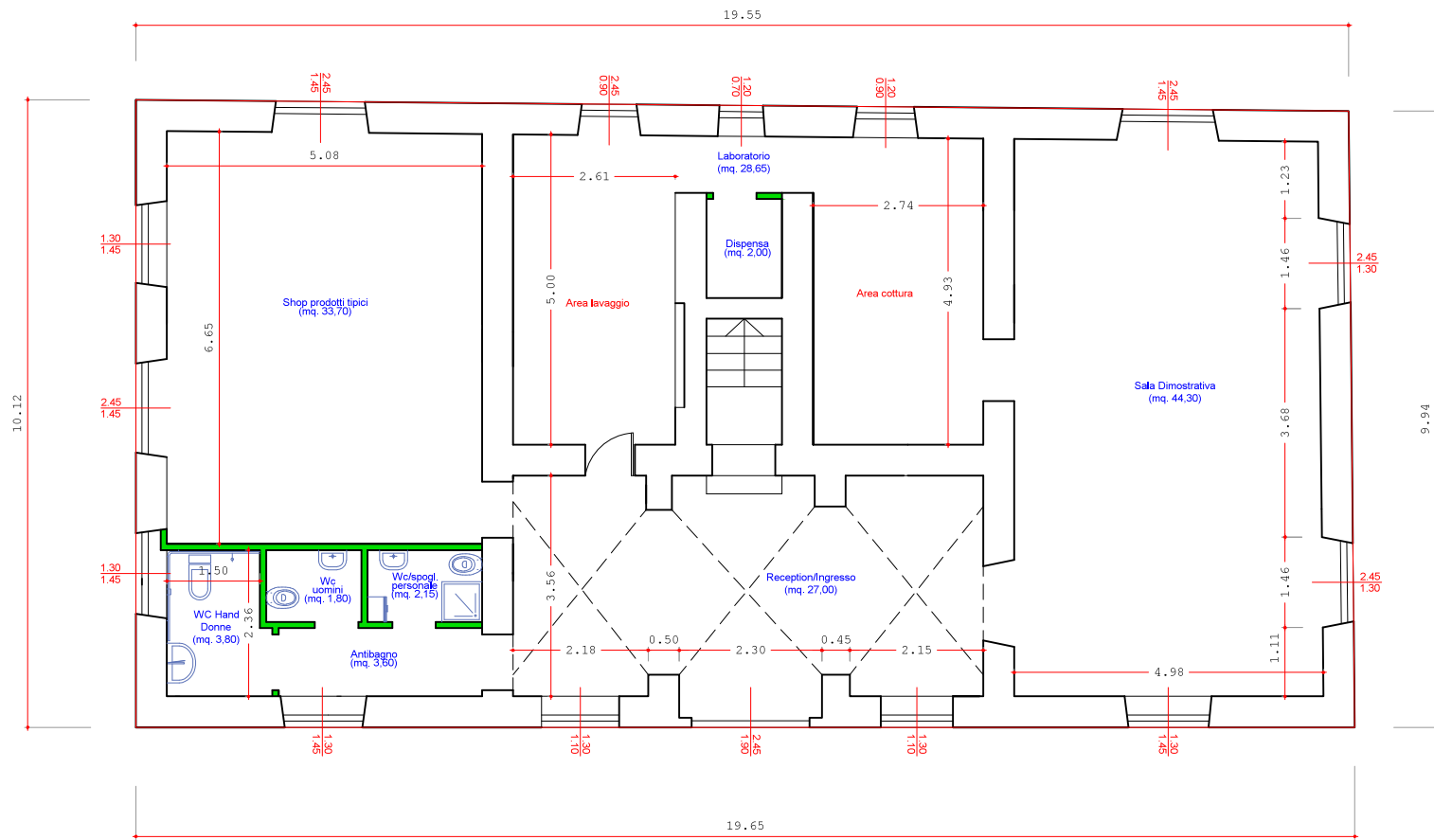
PIANTA PIANO TERRA _ Q.0,05
