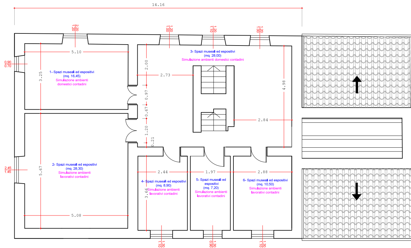
PIANTA PRIMO PIANO _ Q.3,20
